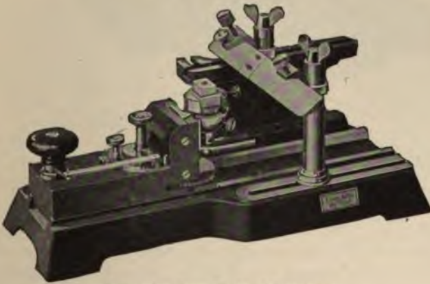
FIG. 36.—Base Sledge Microtome
